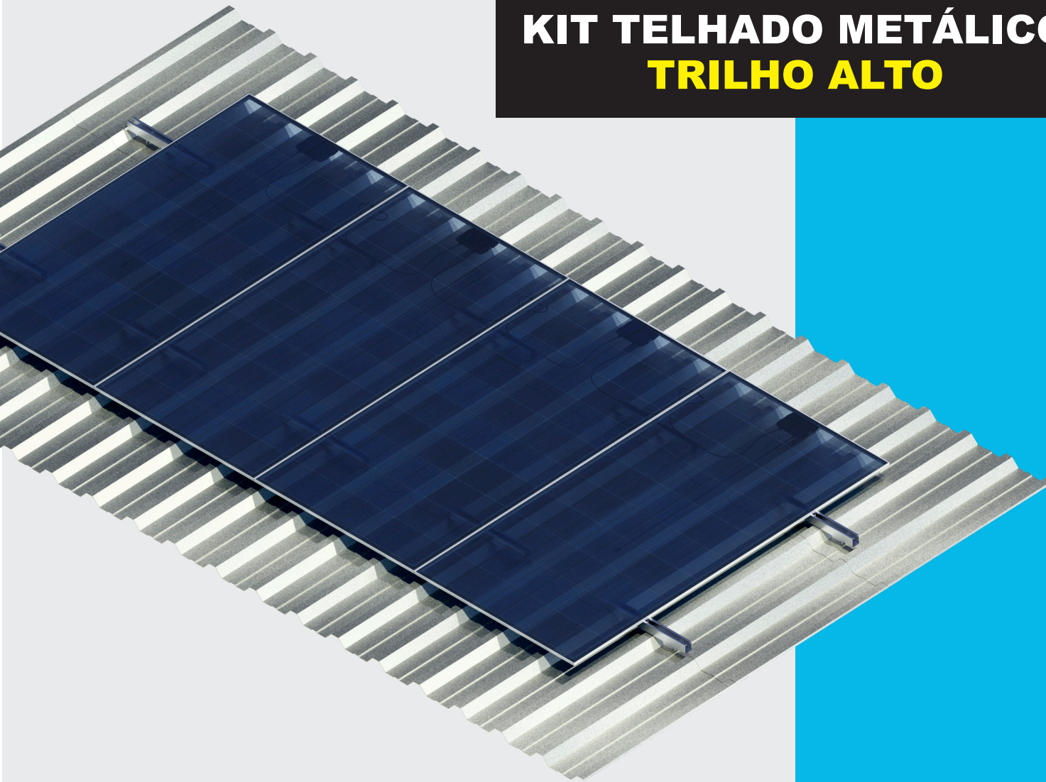
KIT TELHADO METÁLICO TRILHO ALTO 04 MÓDULOS - COMPOSIÇÃO
