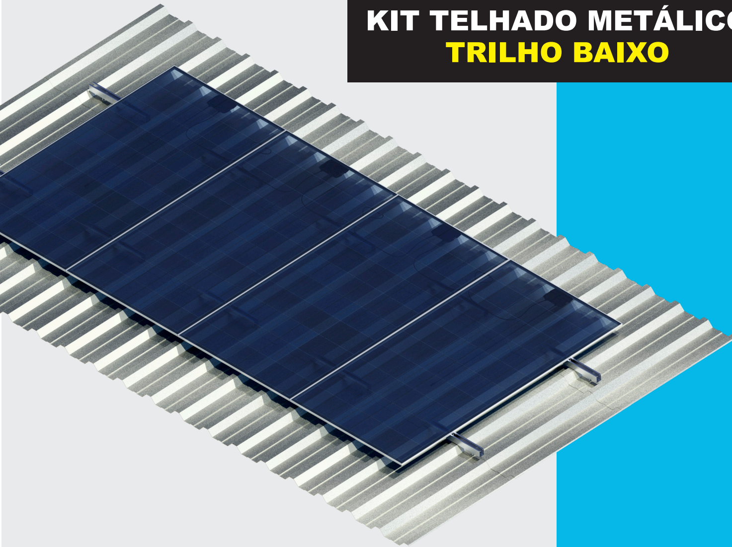
KIT TELHADO METÁLICO TRILHO BAIXO 04 MÓDULOS - COMPOSIÇÃO
